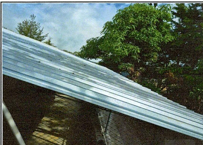
Foto 2: Mejoramiento con estructura tipo pórtico e instalación de lámina troquelada calibre 26 en la cocina.
