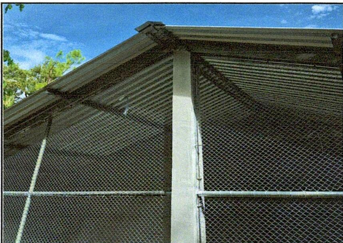
Foto 1: Mejoramiento con estructura tipo pórtico e instalación de lámina troquelada calibre 26 en la cocina.
